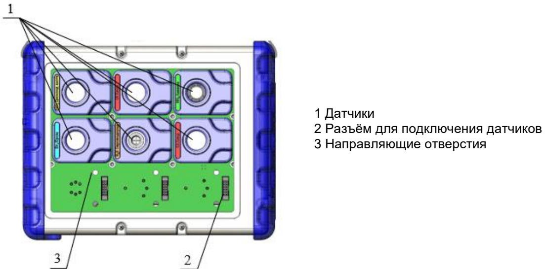
Рисунок 8.1 – Отсек для датчиков с указанием элементов
